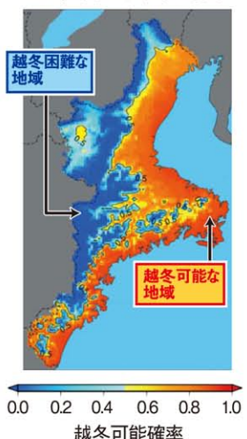
2015年のミナミアオカメムシ越冬可能地域予測図
